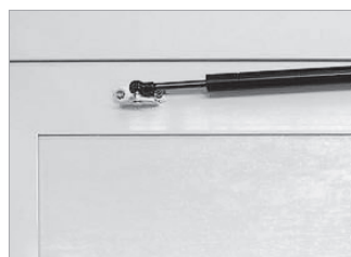
Gasdruckdämpfer zur Endlagensicherung, alternativ Obentürschließer (mit/ ohne Rastfeststellung) erhältlich
